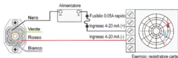
SCHEMA 3: 4-20 mA, collegamento con alimentatore esterno
