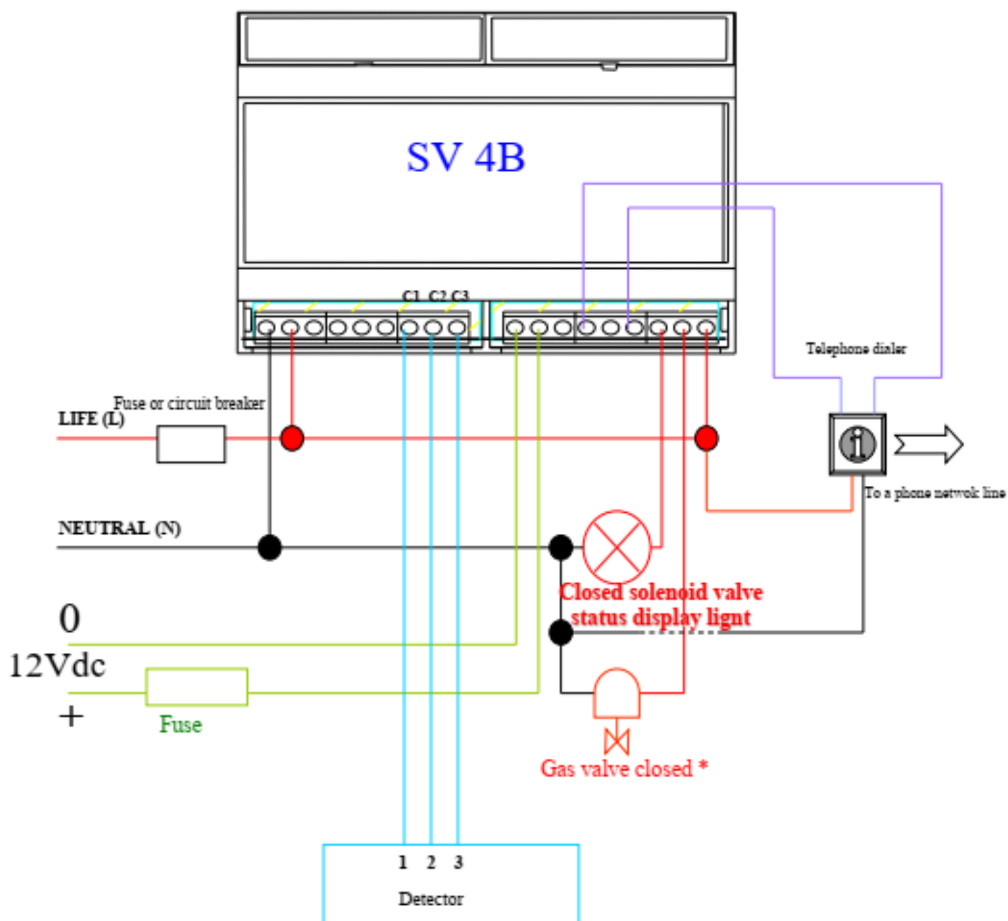
Figure 7: Exemple d'installation d'un Surveyor 4B avec un capteur
