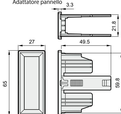
Adattatore pannello
